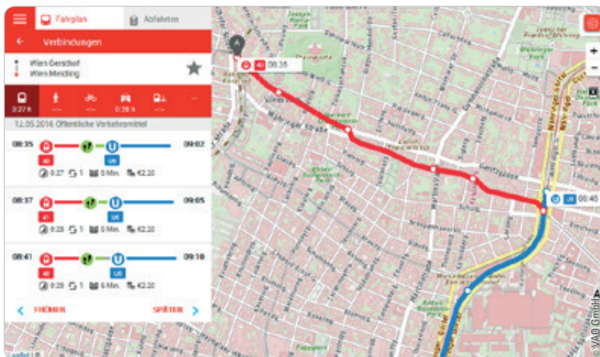
Abbildung 2: Die VAO-Webapplikation
