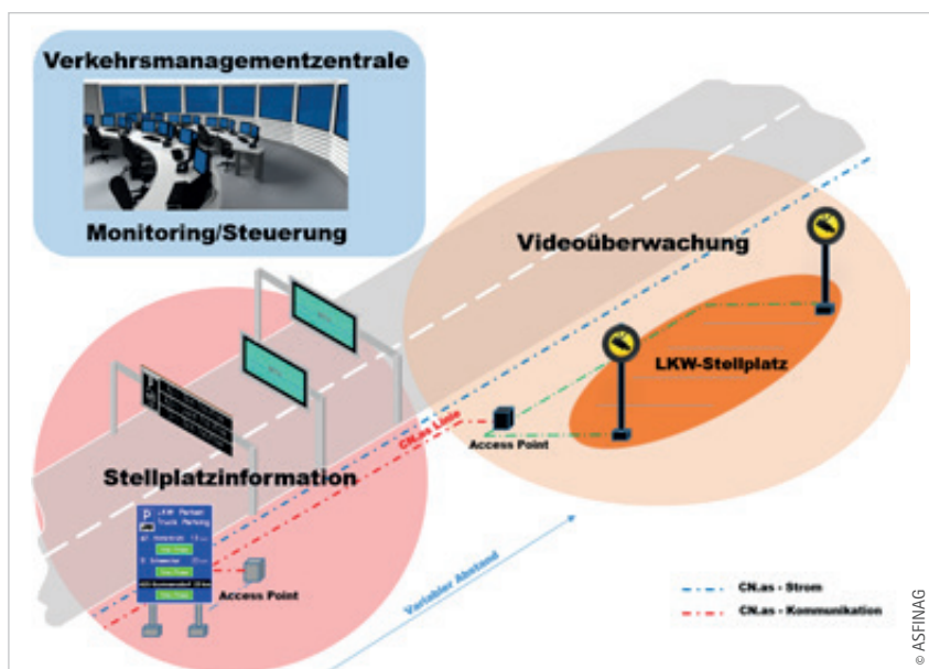
Abbildung 14: Systemstruktur SPIS
